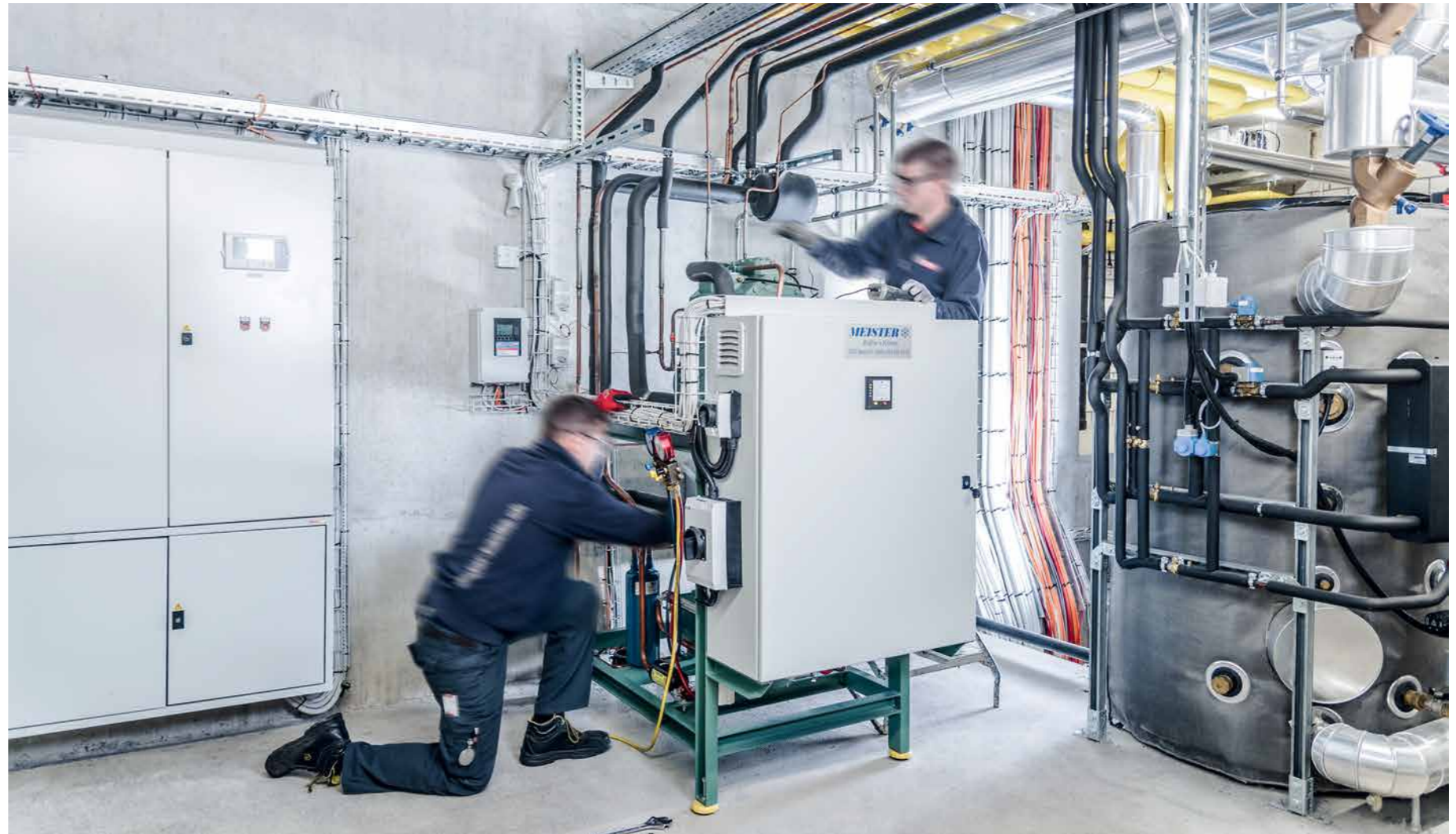
Abb: Maschinenraum einer Kälteanlage
